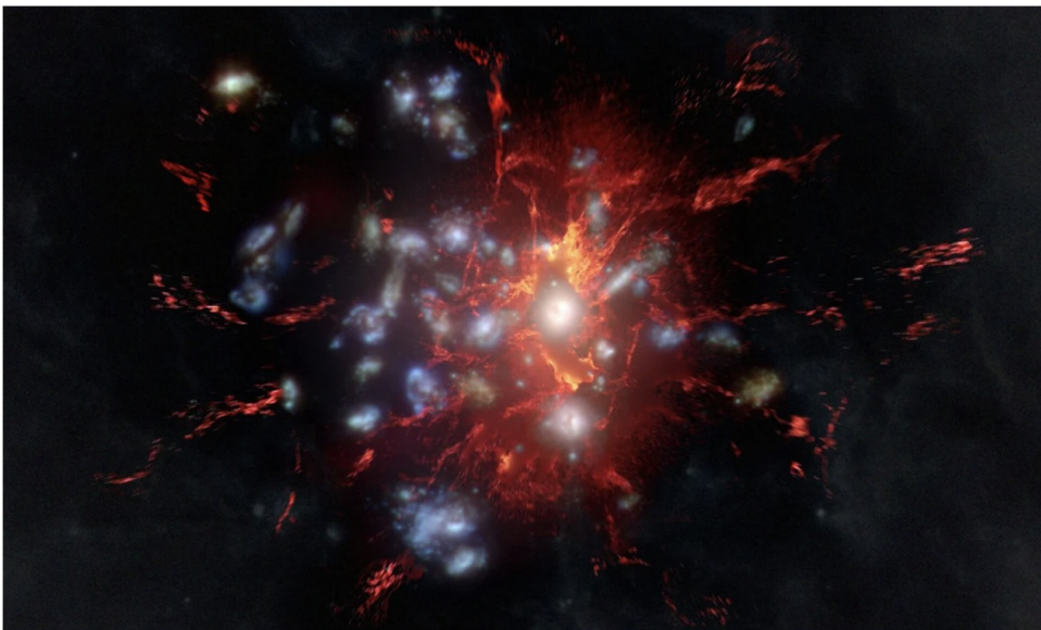
Ilustración del gas molecular distribuido (rojo) que rodea a las galaxias del núcleo del protocúmulo SPT2349–56. Crédito: MPIfR/N.Sulzenauer.
